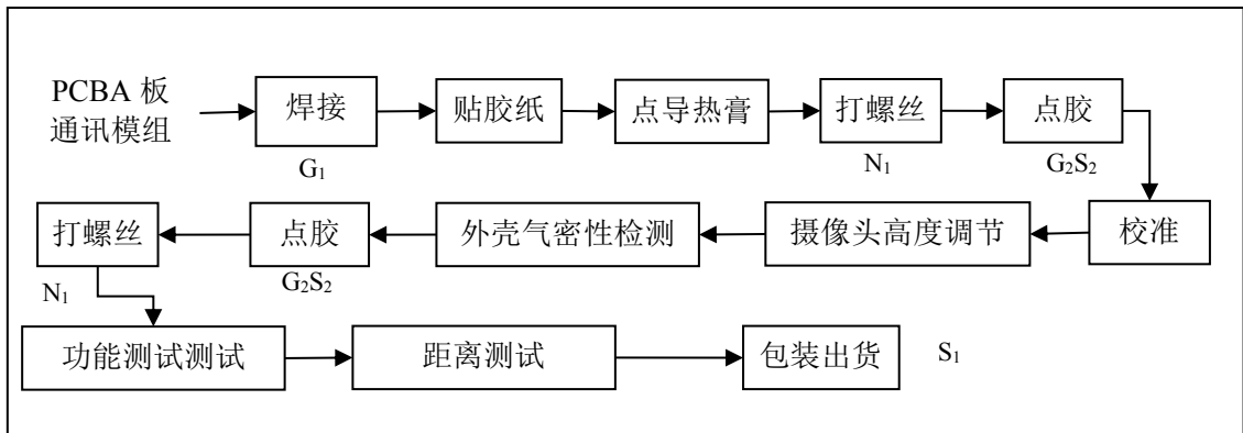
图 2-1 生产工艺流程图
